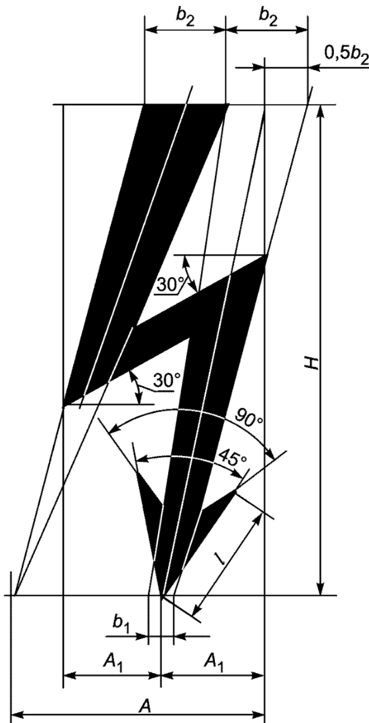
Рисунок Н.1 - Графический символ электрического напряжения
