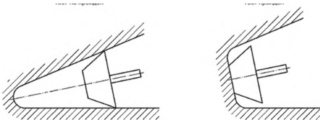
Рисунок 10 — Проверка соответствия оборудования требованиям к обеспечению предотвращения застреваний частей тела
