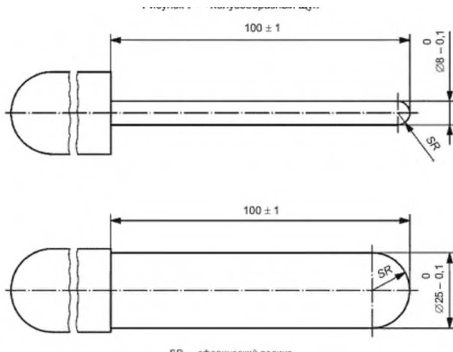
Рисунок 8 — Цилиндрические щупы
