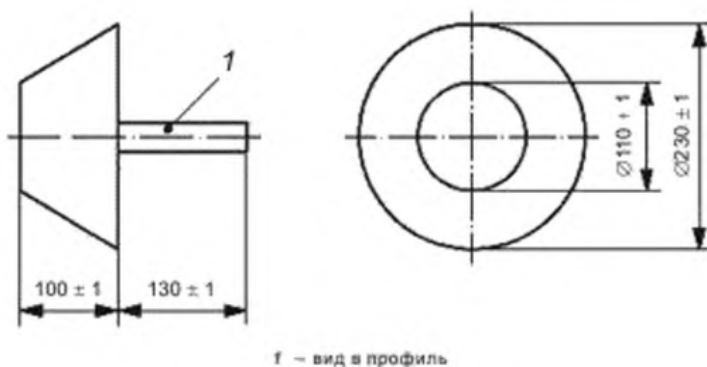
Рисунок 7 — Конусообразный щуп
