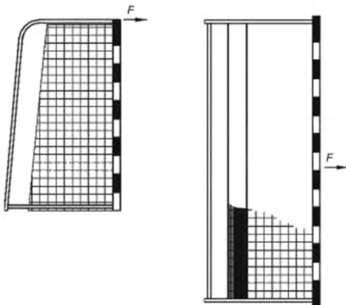
Рисунок 4 — Проверка стабильности ворот для мини-футбола
