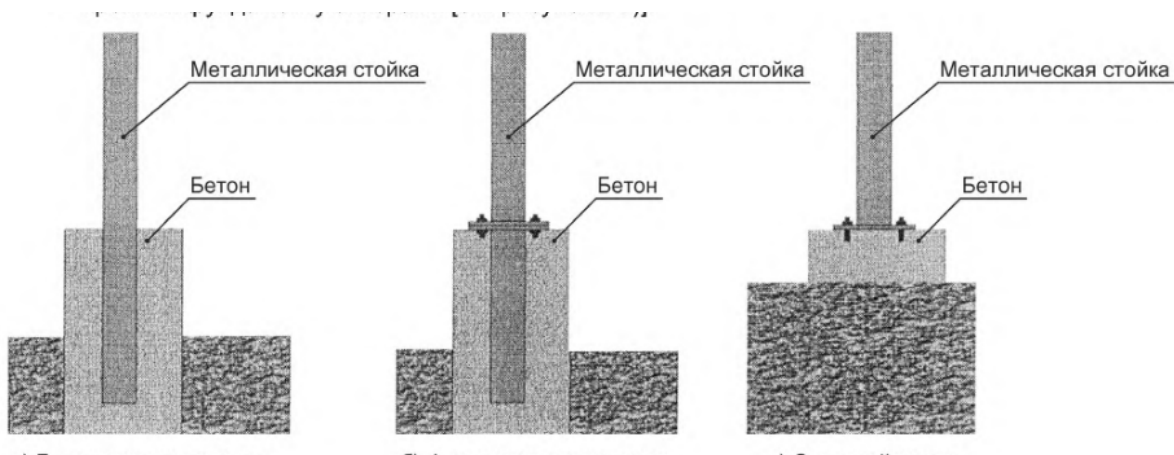
а) Бетонирование опоры б) Фланцевое соединение в) Стальной анкер
