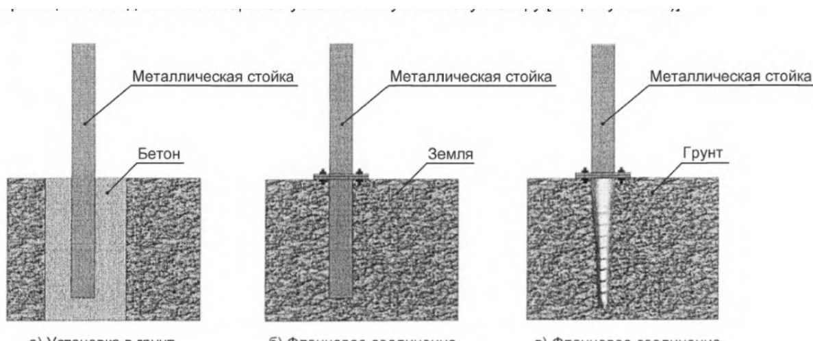
а) Установка в грунт с бетонированием б) Фланцевое соединение к закладной опоре в) Фланцевое соединение к винтовой опоре
