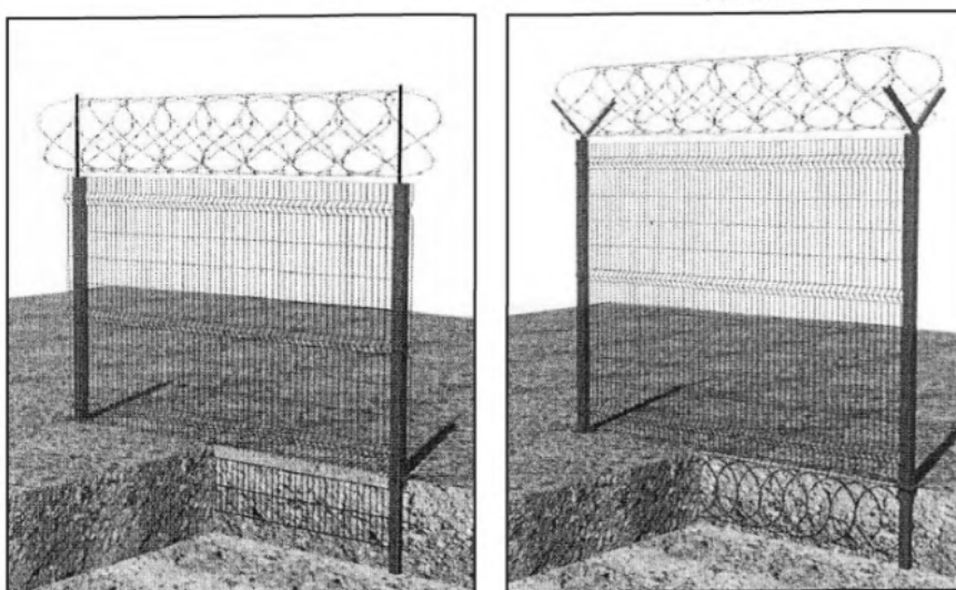
в) Дополнительная сетчатая панель г) Плоский барьер безопасности
