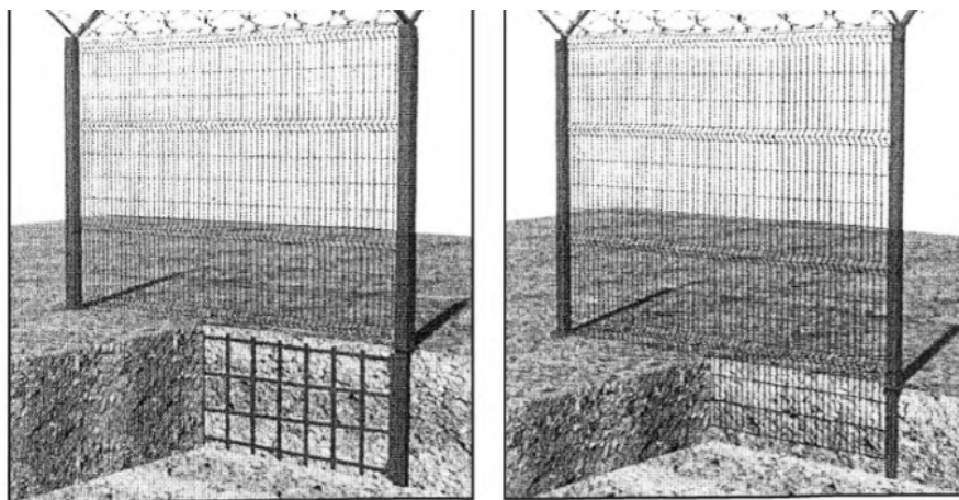
а) Сварная решетка в грунте б) Заглубление сварной сетчатой панели
