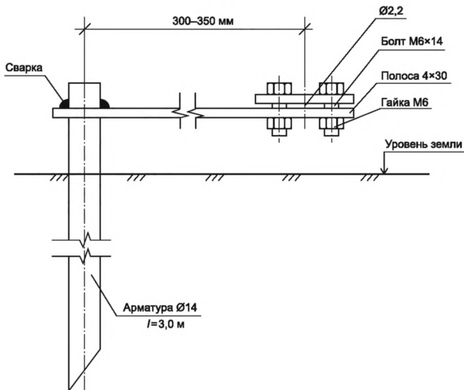
Рисунок Б.1 — Вариант исполнения заземляющего устройства для систем ограждений
