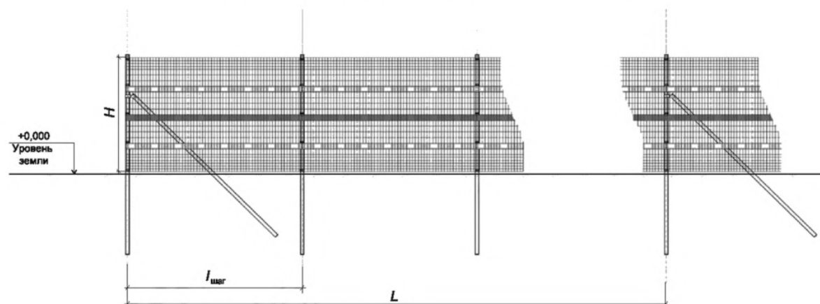
Рисунок 9 — Рулонно-секционное ограждение с типом полотна P1
