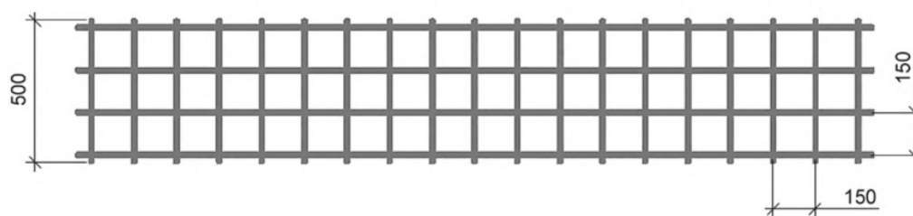
Рисунок 4 — Противоподкопное усиление
