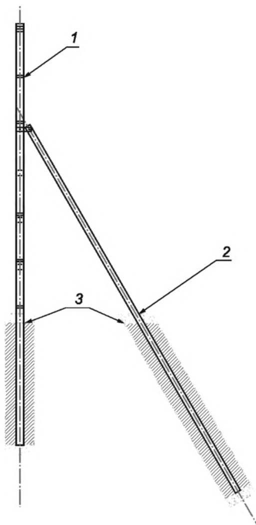
Рисунок 5 — Опора в бетонном фундаменте
