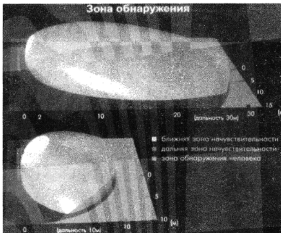
Рисунок 86 - Зоны обнаружения извещателя.
