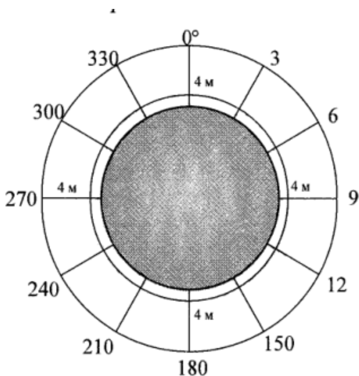
Рисунок 34 — Форма зоны обнаружения ультразвукового извещателя в продольном сечении
