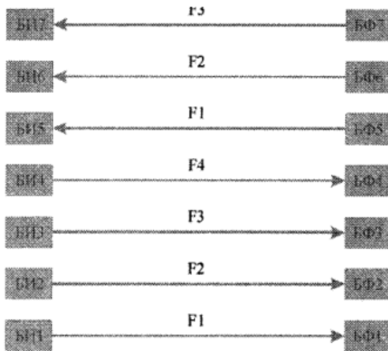
Рисунок 67 — Пример ИК барьера со встречно направленными лучами
