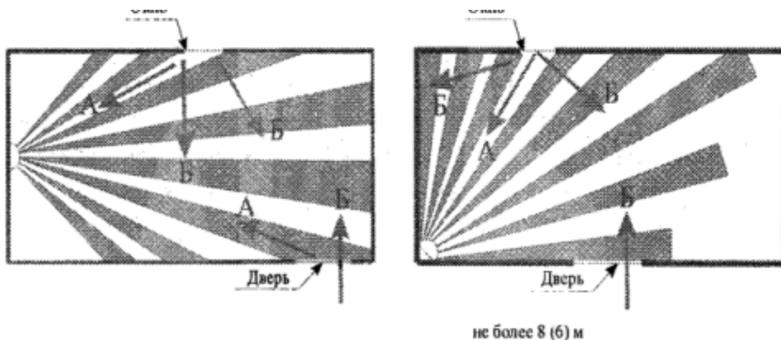
Рисунок 41 — Возможные траектории перемещения нарушителя в зоне обнаружения ИК извещателя, устанавливаемого на стене
