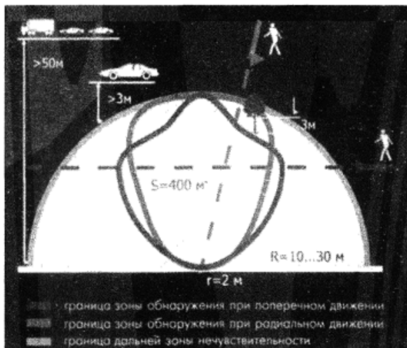
Рисунок 87 - Обнаружение при перемещениях по любым траекториям
