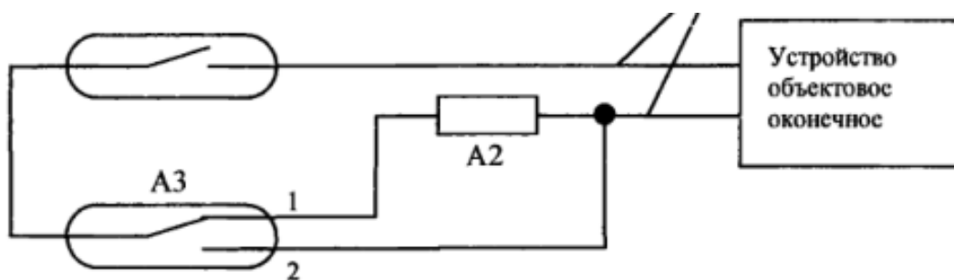
Рисунок 9 — Схема защиты магнитоcontactного извещателя от саботажа
