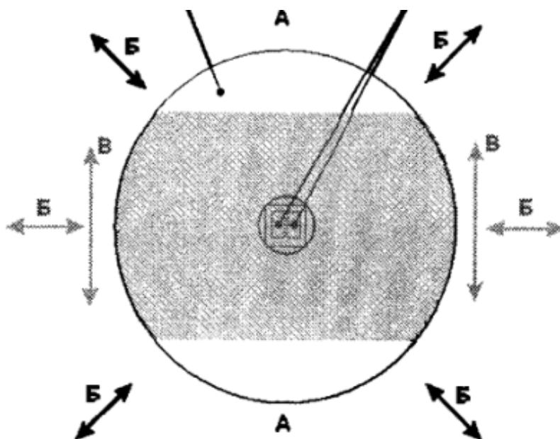
Рисунок 42 — Возможные траектории перемещения нарушителя в зоне обнаружения ИК извещателя, устанавливаемого на потолке
