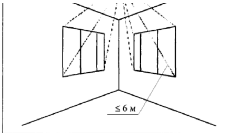
Рисунок 19 – На потолке (вариант 2)
