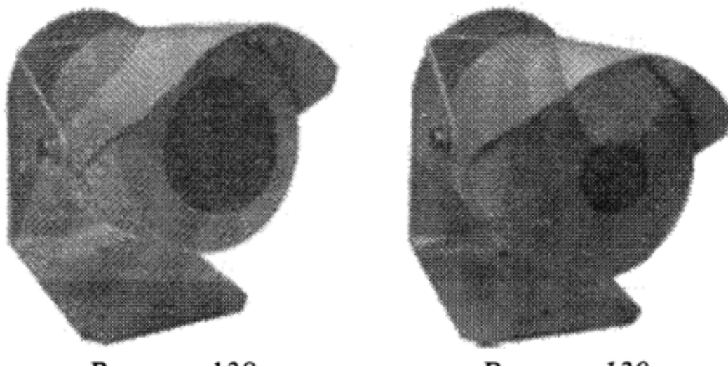
Рисунок 138 Рисунок 139 Извещатель «ИПП-Ех» Извещатель «ИПП-Ех исп. 1» Основные технические характеристики извещателя «ИПД-Ех» приведены в таблице 45.
