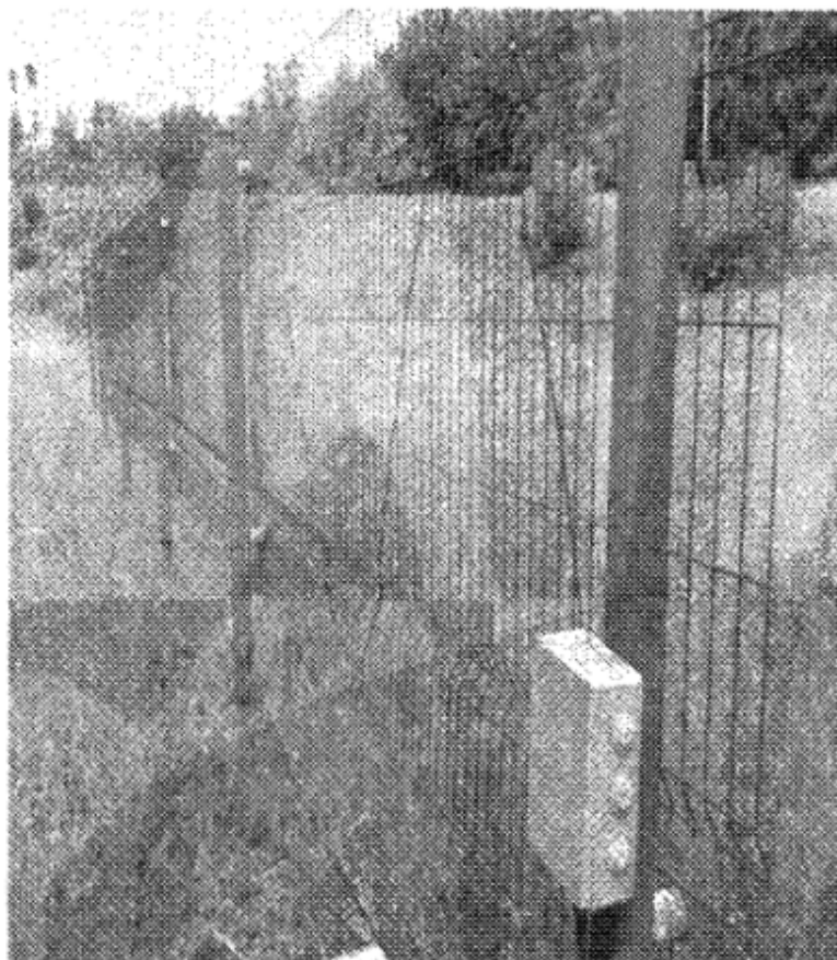
Рисунок 119 — Пример установки извещателя «Рубеж» на металлическом ограждении
