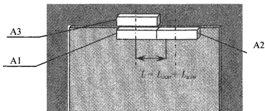
Рисунок 11 - Схема размещения мест монтажа извещателя иДВМП
