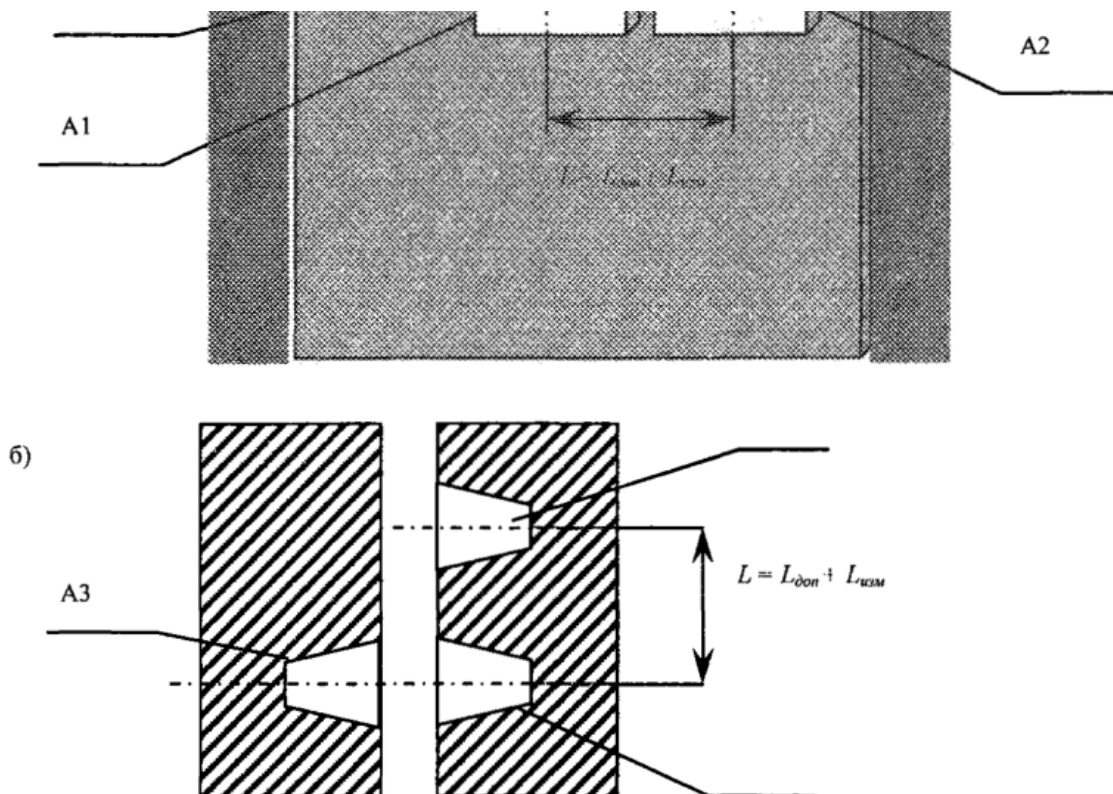
Рисунок 10 — Схема размещения мест монтажа извещателя и ДВМП
