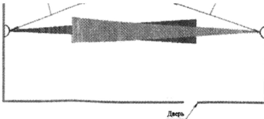
Рисунок 106— Установка извещателей с поверхностной зоной обнаружения в помещении длиной более 10 м
