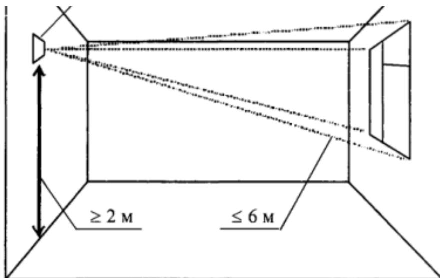
Рисунок 17-Н а противоположной стене
