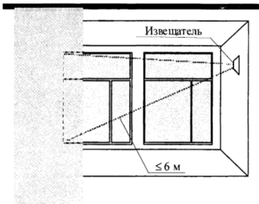
Рисунок 15 — Между стеклом и жалюзи
