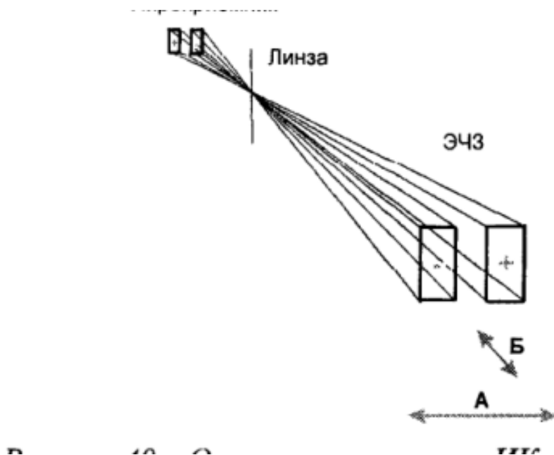
Рисунок 40 — Оптическая система ИК извещателя
