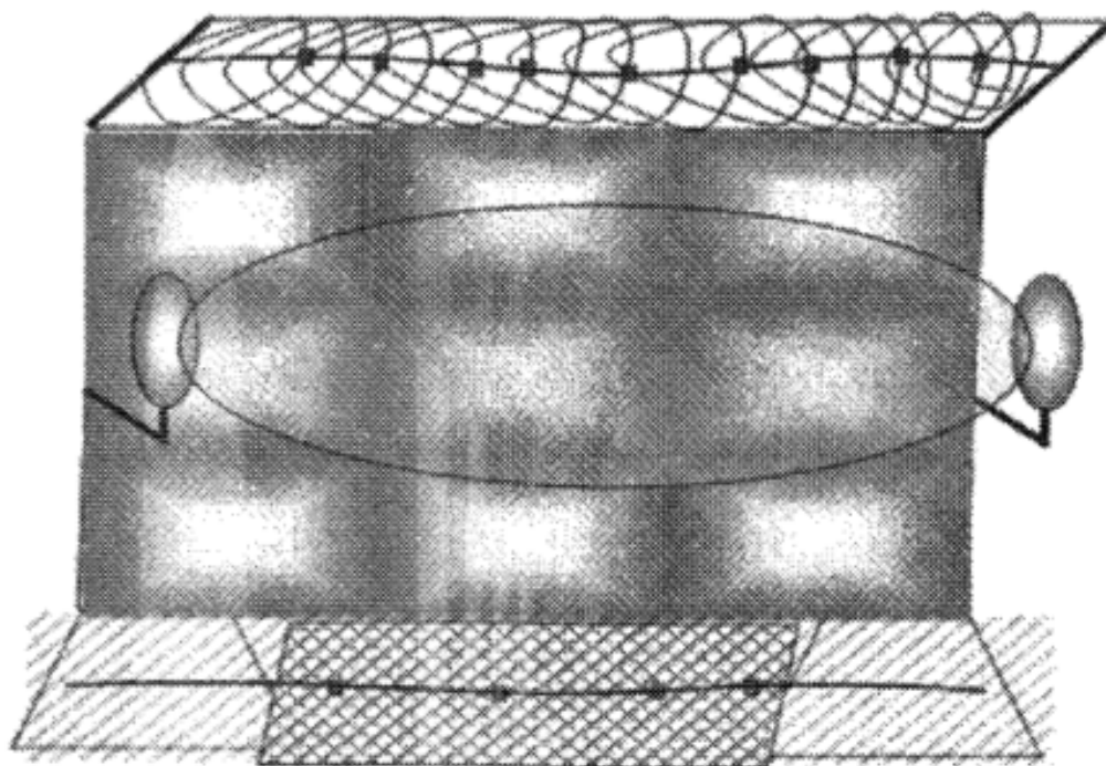
Рисунок 120 — Установка извещателя «Рубеж» на бетонном заграждении
