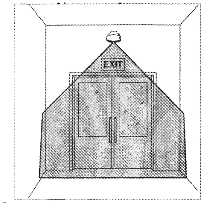
Рисунок 109 — Установка извещателя с поверхностной зоной обнаружения на стену в плоскости проема
