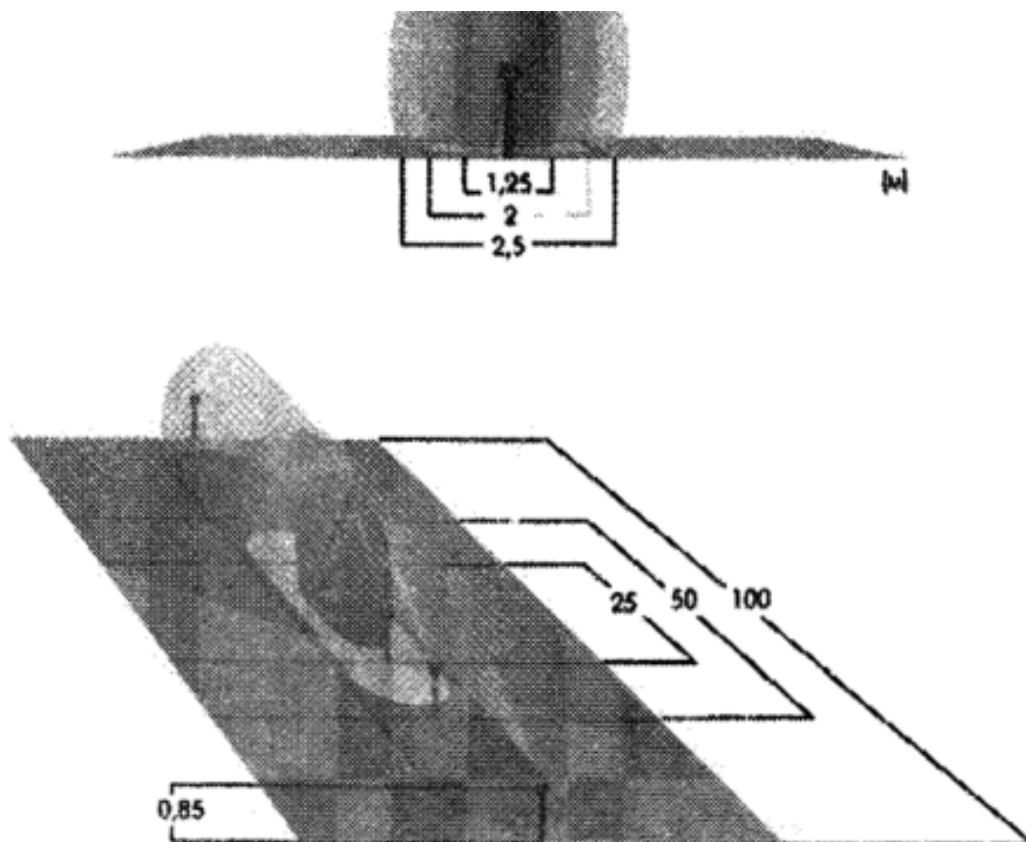
Рисунок 92 - Зоны обнаружения извещателя «Линар-200»
