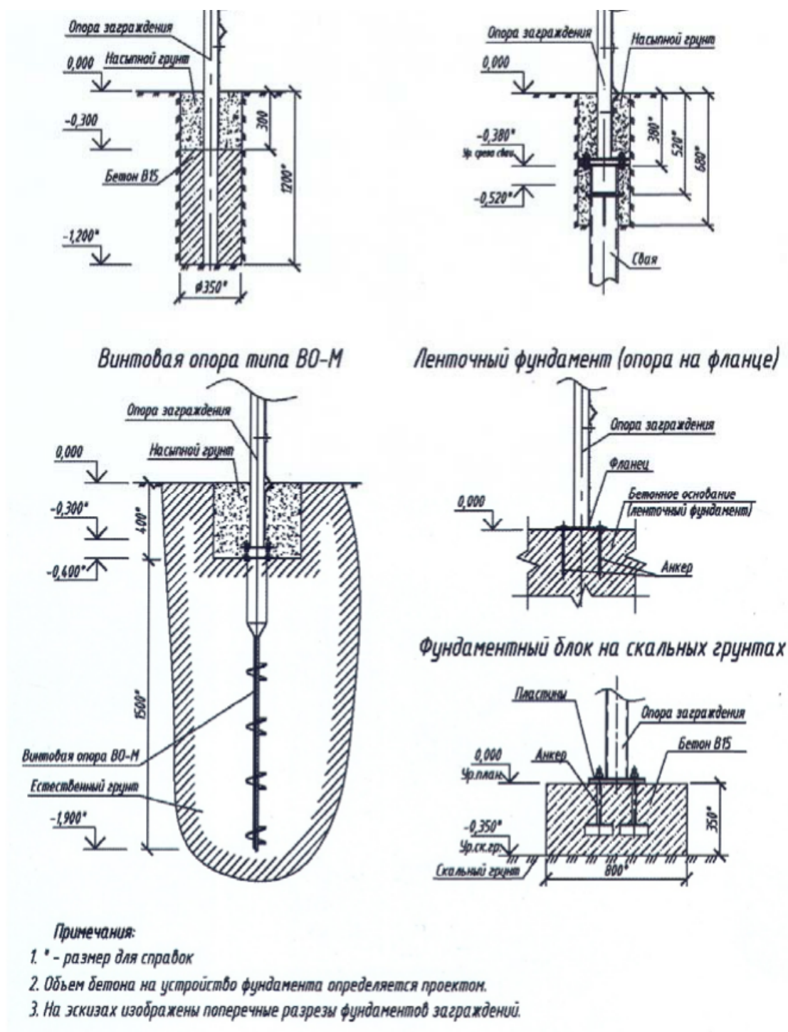
Рис. 2.8. Примеры фундаментов и способы установки опор
