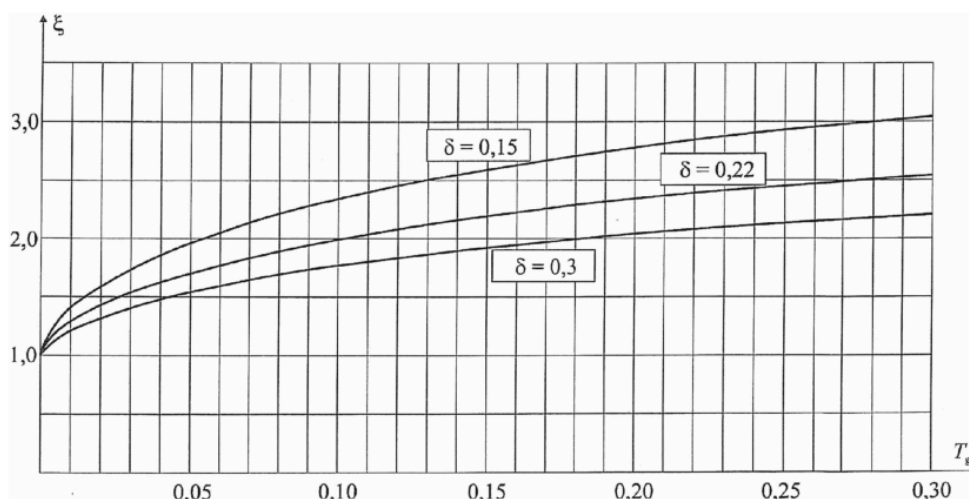
Рисунок 11.1 - Коэффициенты динамичности
