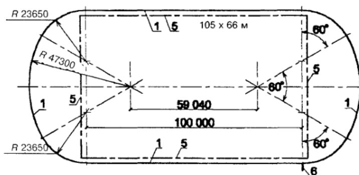
В. ДОРОЖКА ДЛИНОЙ 333,33 м ПРИ ОДНОЦЕНТРОВЫХ ПОВОРОТАХ С РАДИУСОМ 36
