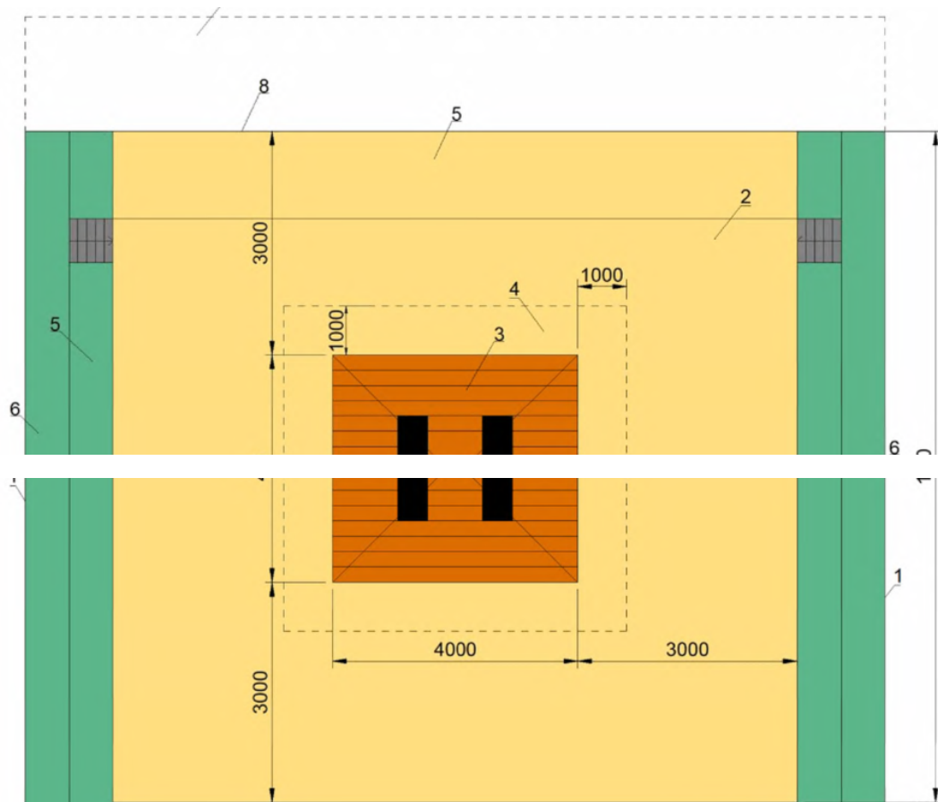
Рисунок Г.25 - Спортивная зона для самбо
