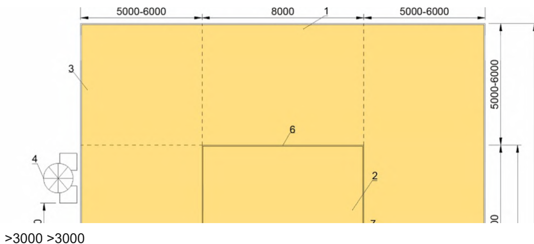
Рисунок Г.29 — Спортивная зона для фехтования на колясках
