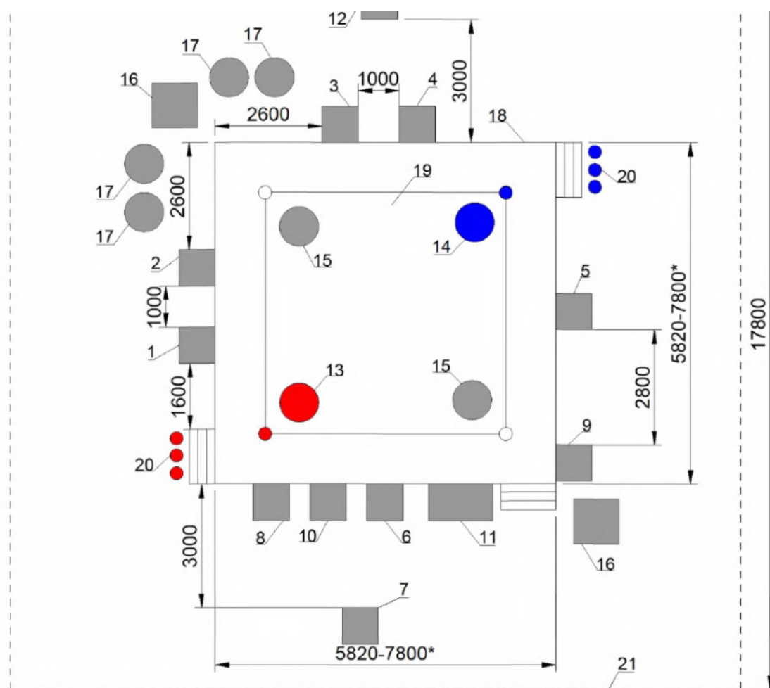
Рисунок Г.21 - Спортивная зона для художественной гимнастики
