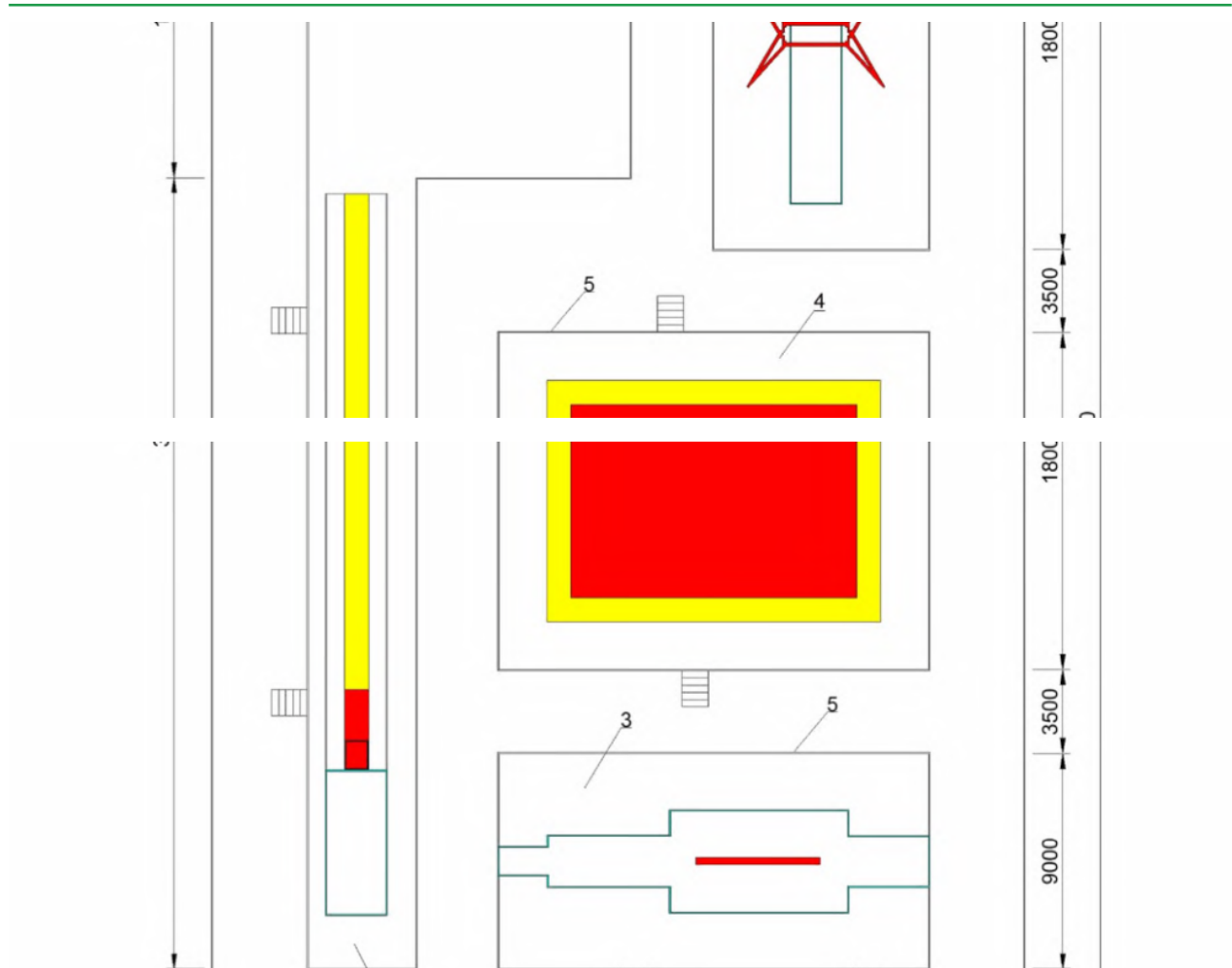
1 - зона опорного прыжка; 2 - зона упражнений на разновысоких брусьях; 3 - зона снаряда «бревно»; 4 - площадка для вольных упражнений; 5 - помост / граница зоны безопасности Рисунок Г.19, лист 2 - Спортивная зона для спортивной гимнастики (женщины)
