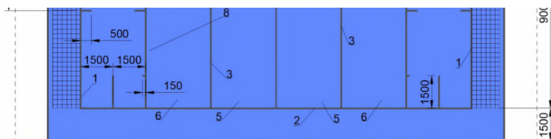
Рисунок Г. 14 - Спортивная зона и разметка для волейбола сидя
