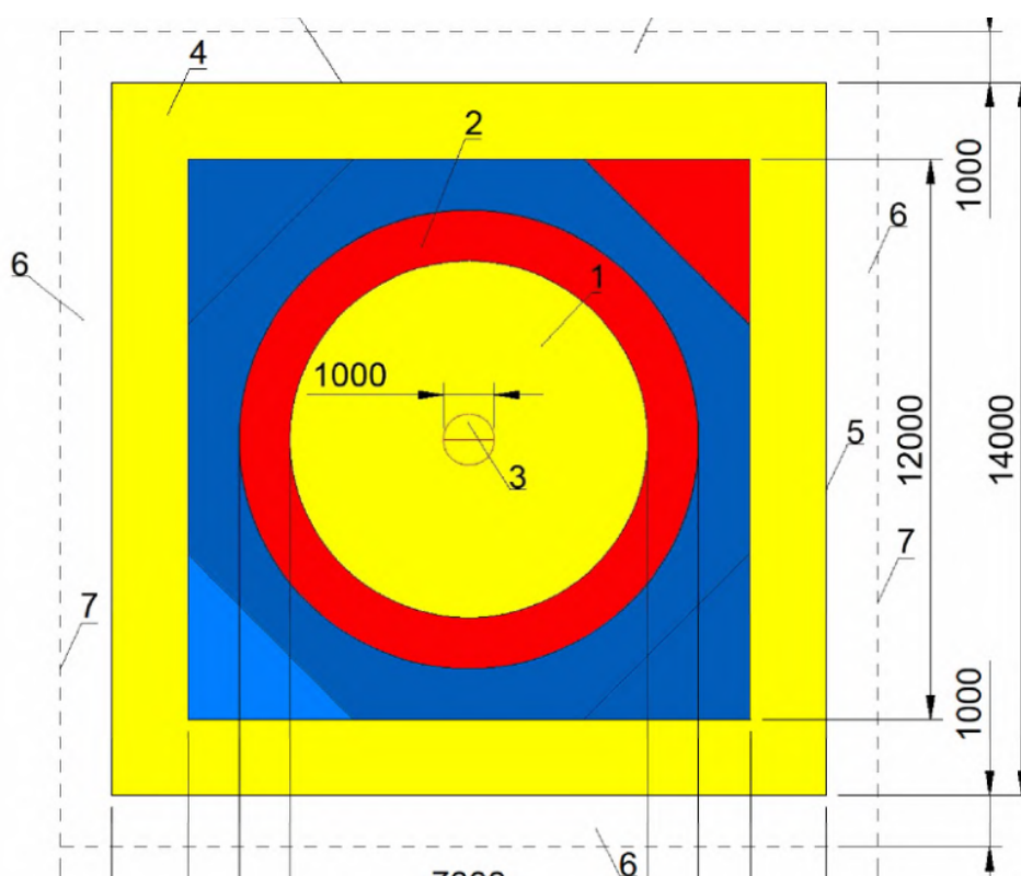
1 - рабочая зона ковра; 2 - зона пассивности; 3 - центр ковра; 4 - зона безопасности; 5 - граница площадки (помоста); 6 - зона размещения судей и обслуживающего персонала; 7 - граница спортивной зоны
