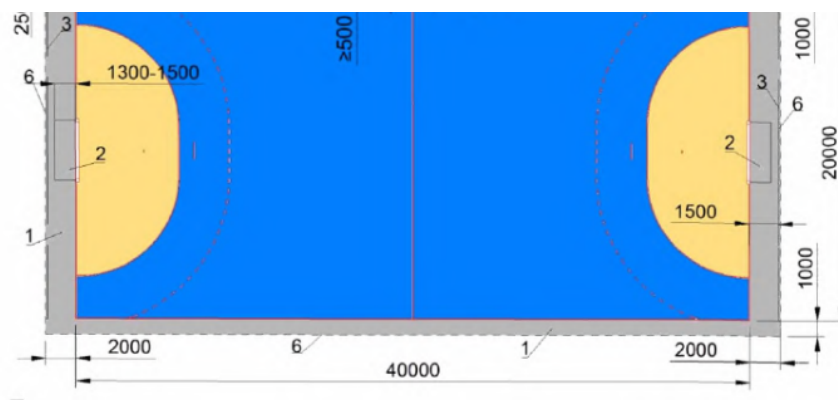
Рисунок Г. 8 - Спортивная зона для волейбола
