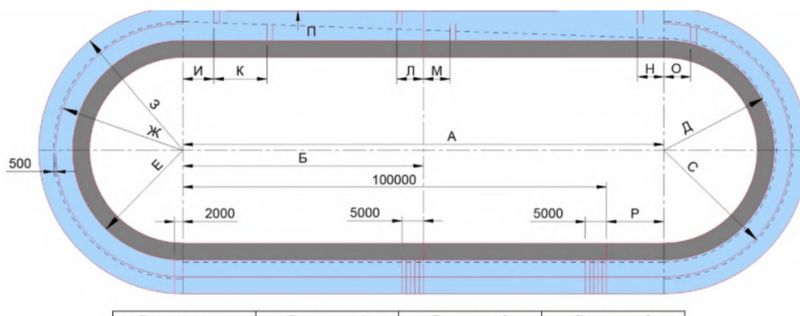
Рисунок Г.1, лист 1 - Спортивная зона для конькобежного спорта
