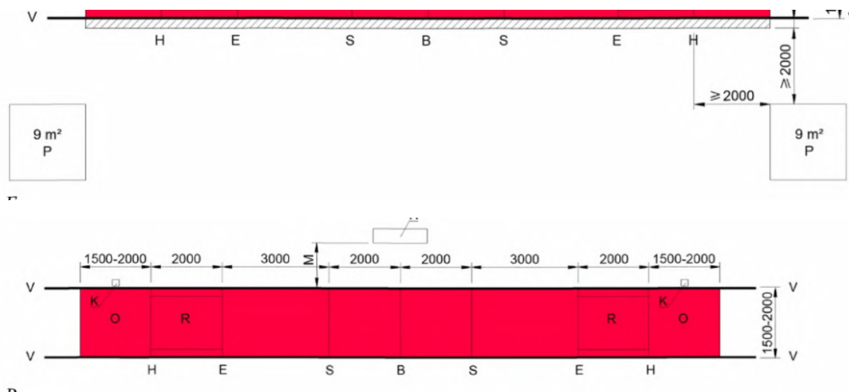
Рисунок Г.26 - Спортивная зона для тяжелой атлетики
